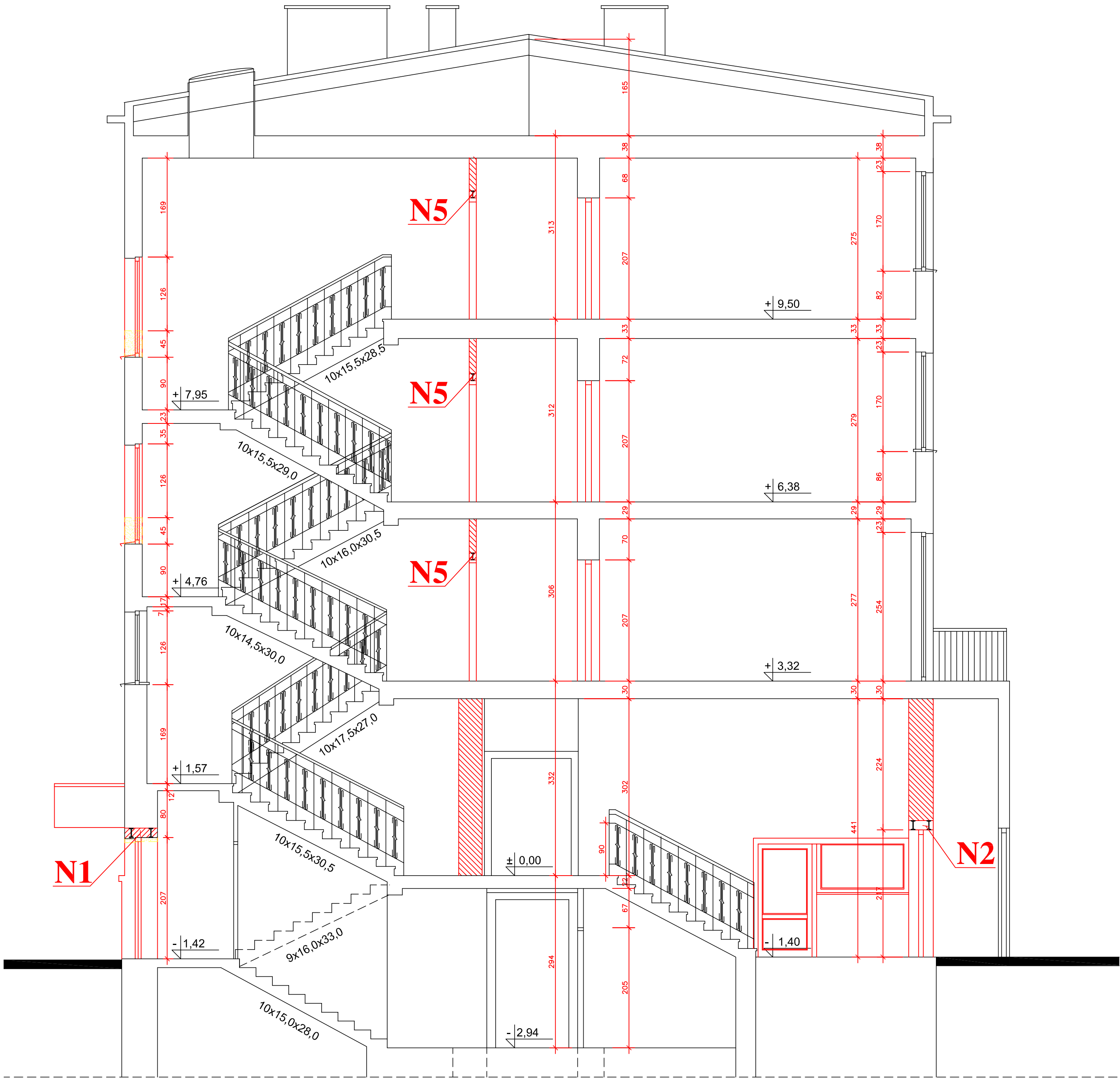
PRZEKRÓJ A-A skala 1:50
