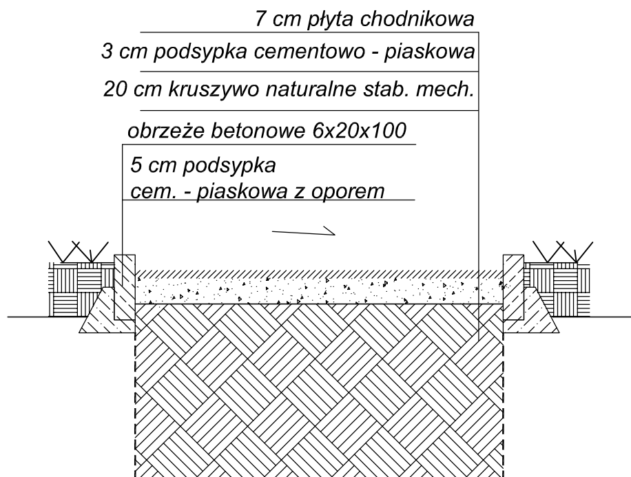
Konstrukcja nawierzchni chodnika i placyków
