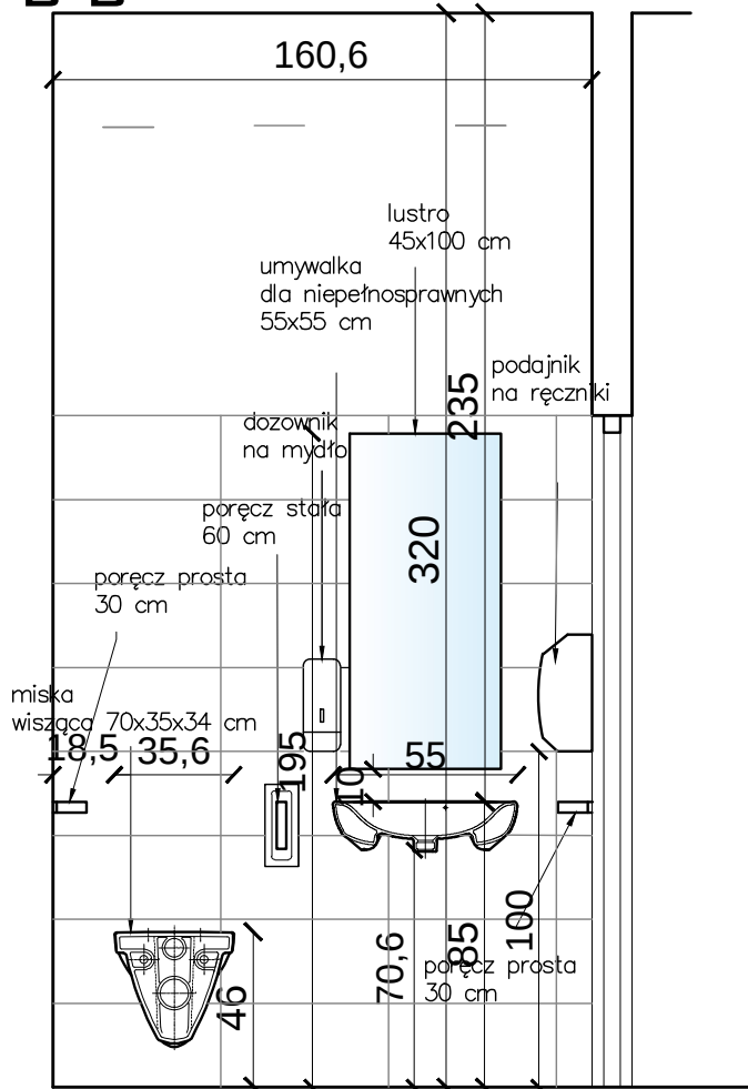
WIDOK B-B
