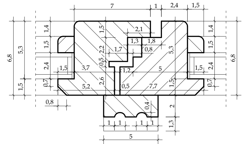
SZCZEGÓŁ "b"
