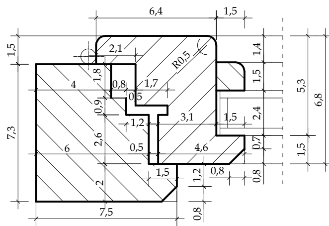
SZCZEGÓŁ "a"
