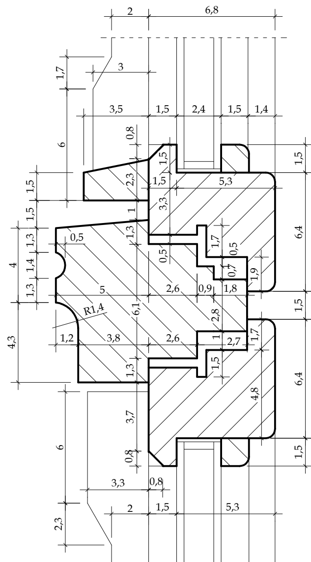
SZCZEGÓŁ "c"
