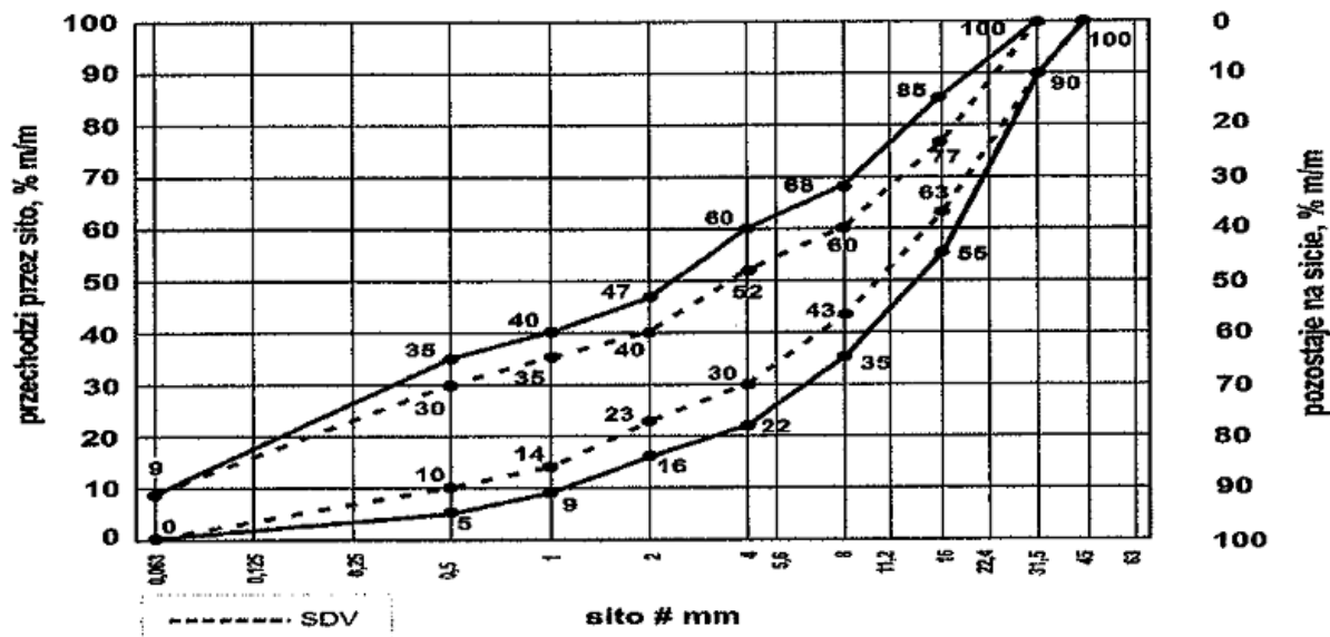
Rysunek 1 Mieszanka niezwiązana 0/31,5 do warstw podbudowy pomocniczej i zasadniczej
